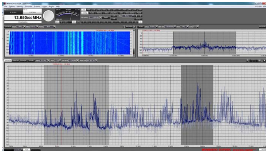
Abb. 1: Die virtuelle Frontplatte des Excelsior zeigt drei große Fenster.
