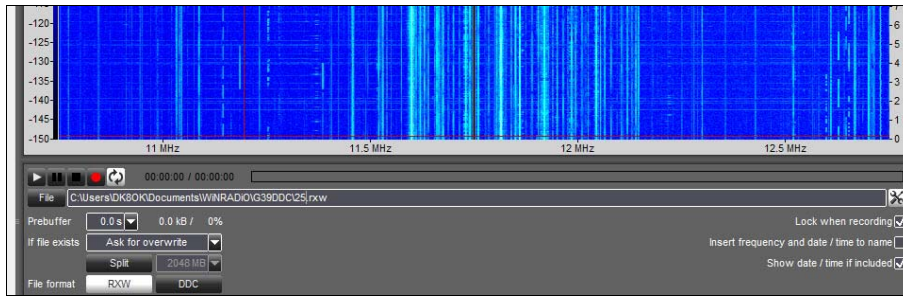
Abb. 5: Für die Aufnahme stehen die Formate "RXW" oder "DDC" zur Verfügung. Ist das Kästchen "Insert frequency and date/time to name" angeklickt, so wird der gewählte Dateiname um die Mittenfrequenz sowie die Start-Uhrzeit erweitert.
