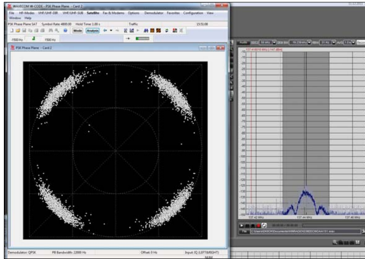
Abb. 17: Links die saubere Darstellung der Vierphasenmodulation des ORBCOMM-Signals mit dem W-Code von Wavecom, rechts die Darstellung des Signals als Spektrum beim Excelsior.
