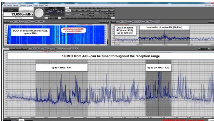
Abb. 2: Das untere Fenster zeigt insgesamt den aktiven Bereich des Analog-/Digitalwandlers von 16 MHz Breite. Innerhalb dieses Bandes sind zwei Empfänger aktiv: RX1 mit 4 MHz Bandbreite und RX2 mit (hier) 2 MHz Bandbreite. Im Fenster oben links ist das Sonogramm von RX2 zu sehen, in der Mitte die Bandbreite des Demodulators (10kHz) Das Fenster oben rechts zeigt den Ausgang des DDC2 zwischen 20 (hier) und 320 kHz.
