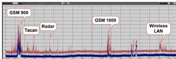
Abb. 13: Ein Sweep über fast zwei Gigahertz (800 MHz – 2,6 GHz) zeigt die Belegung in diesem Bereich – einige herausgehobene Beispiele sind markiert.
