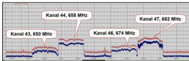
Abb. 15: Via „Sweep“ lassen sich auch alle DB-TV-Kanäle in einer Gegend schnell apportieren; hier eine herausvergrößerte Ansicht aus dem UHF-Band IV und V.
