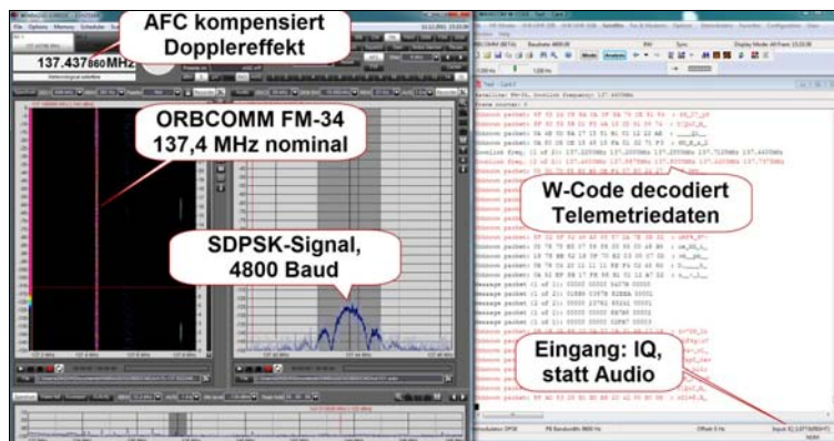
Abb. 16: Empfang eines der 36 umlaufenden ORBCOMM-Satelliten auf 137,4 MHz und die Decodierung der Telemetriedaten.
