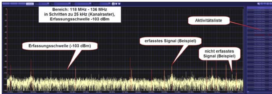
Abb. 10: Alles ist vorbereitet, um ein Aktivitätsmuster im Flugfunkband von 118 bis 136 MHz zu erstellen. Danach wurde der Suchlauf gestartet.
