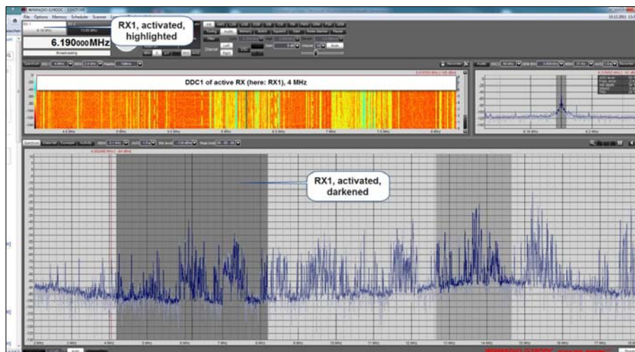
Abb. 3: Schaltet man von RX2 auf RX1, so wechselt das Fenster oben links von 2 MHz zu 4 MHz Bandbreite. Zugleich erscheint im unteren Fenster nun RX1 abgedunkelt, statt in Abbildung 2 der RX2. Des Weiteren habe ich hier die Bandbreite DDC2 von 20 kHz auf 50 kHz erweitert – Fenster oben rechts. So zeigt sich noch mehr von der Umgebung des Signals.
