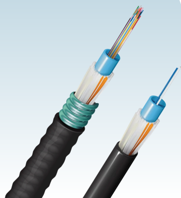
Glasfaserkabel
