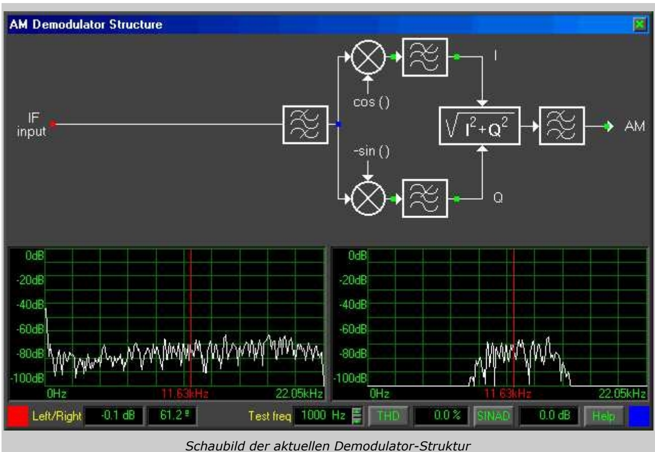
Schaubild der aktuellen Demodulator-Struktur
